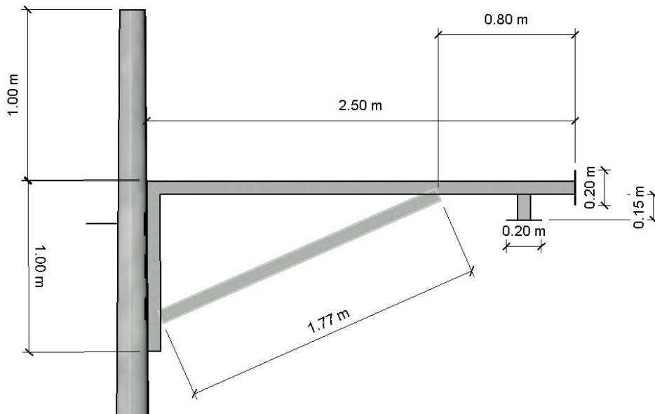
Ilustración 1: Dimensiones de Brazo tipo L de 2.5 m de longitud
