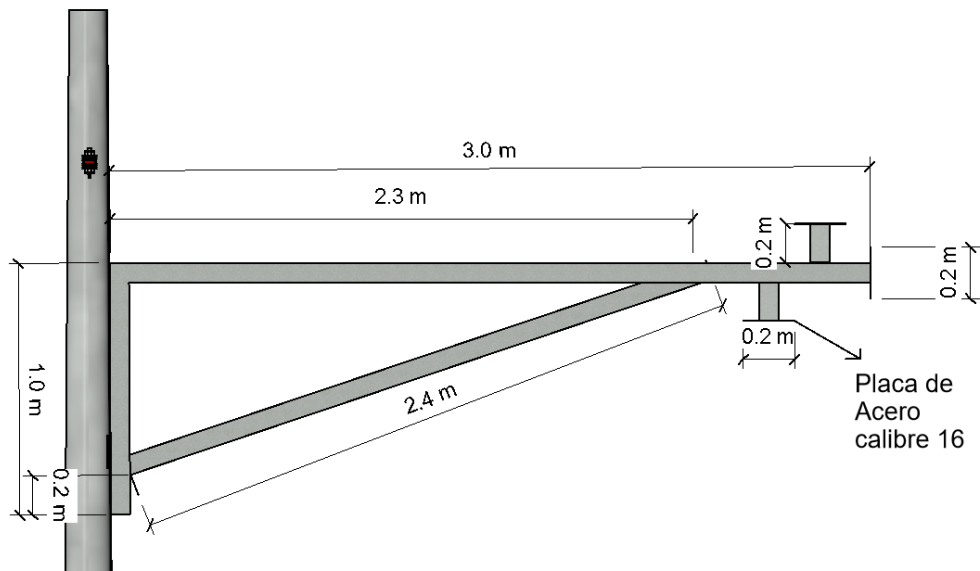
Ilustración 2: Dimensiones de Brazo tipo L de 3.0 m de longitud
