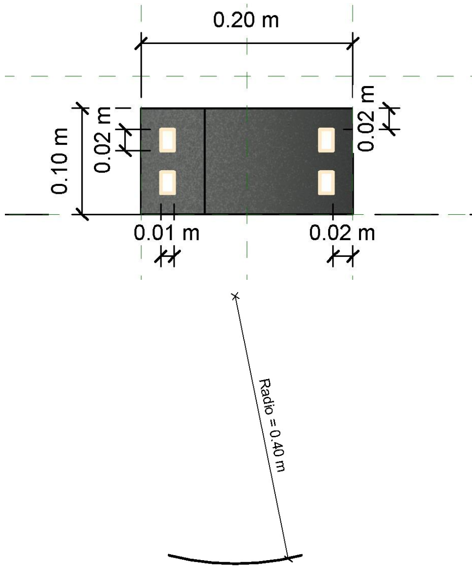
Ilustración 7: Detalles de placas metálicas de sujeción a poste de brazo curvo y tipo L
