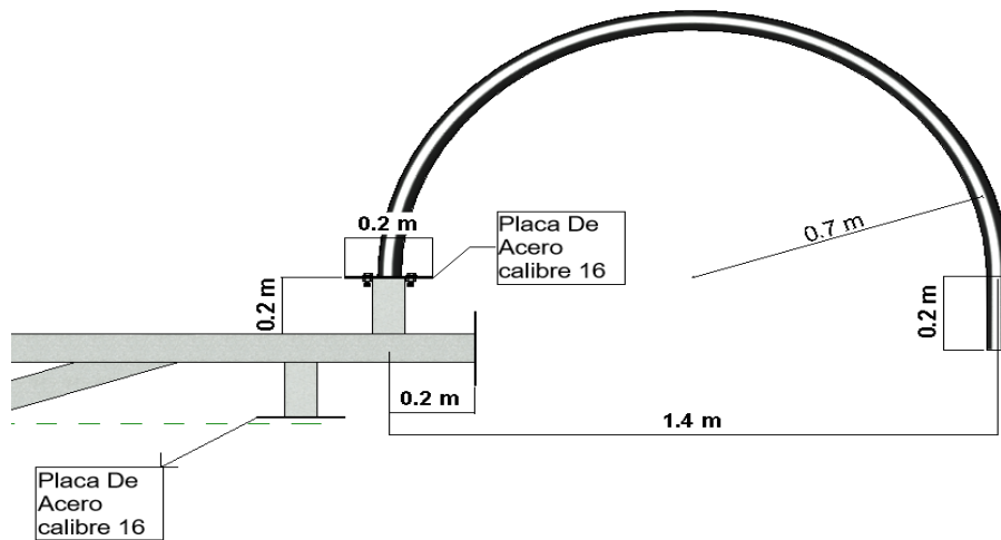
Ilustración 5: Accesorio Tubo Curvo para cámara PTZ
