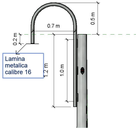
Ilustración 4: Dimensiones de brazo curvo tipo cuello de ganso
