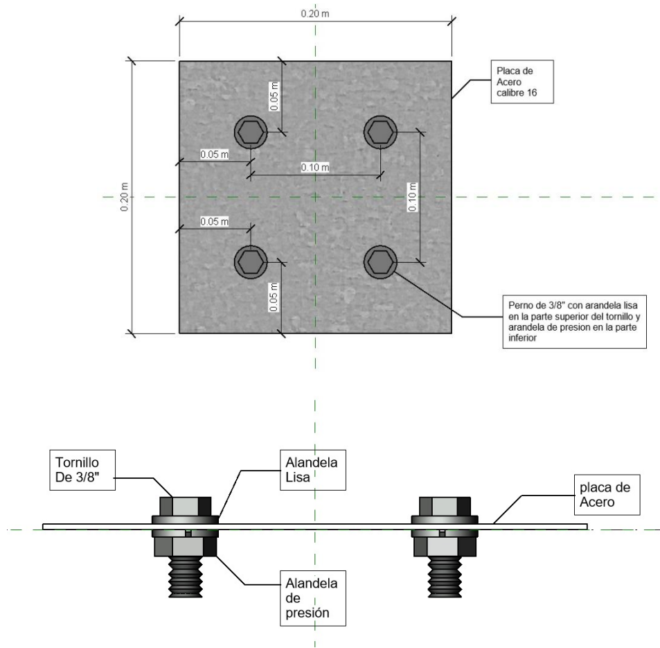
Ilustración 6: Detalles de Placa de Acero
