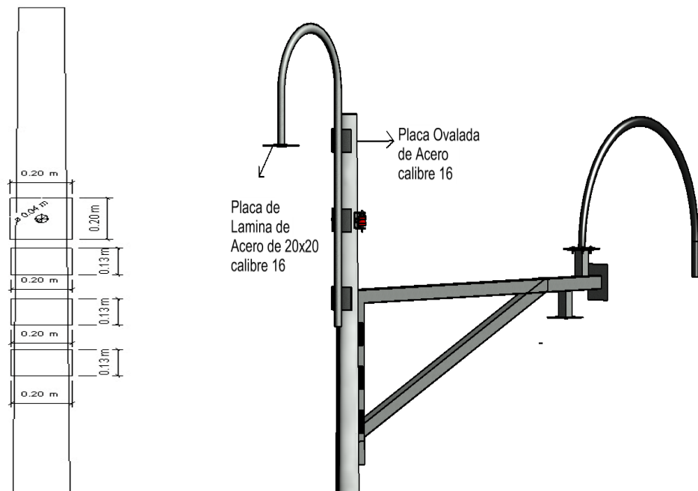
Ilustración 3: Detalles de placas metálicas de sujeción a poste de brazo curvo y tipo L
